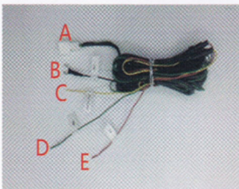
Pripojovací kábel A. Pripojte konektor A komunikačného kábla B. GND (krajina) C napájanie 12V D. Pripojte po kábli zadnej rukoväte E. Pripojte ku káblu ACC (zapaľovanie).
